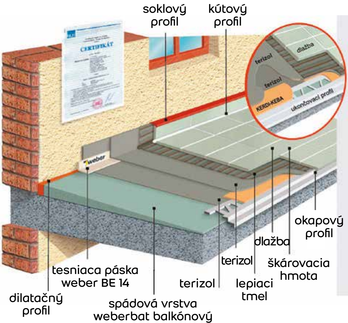
Riešenie A – so spádovým betónom
