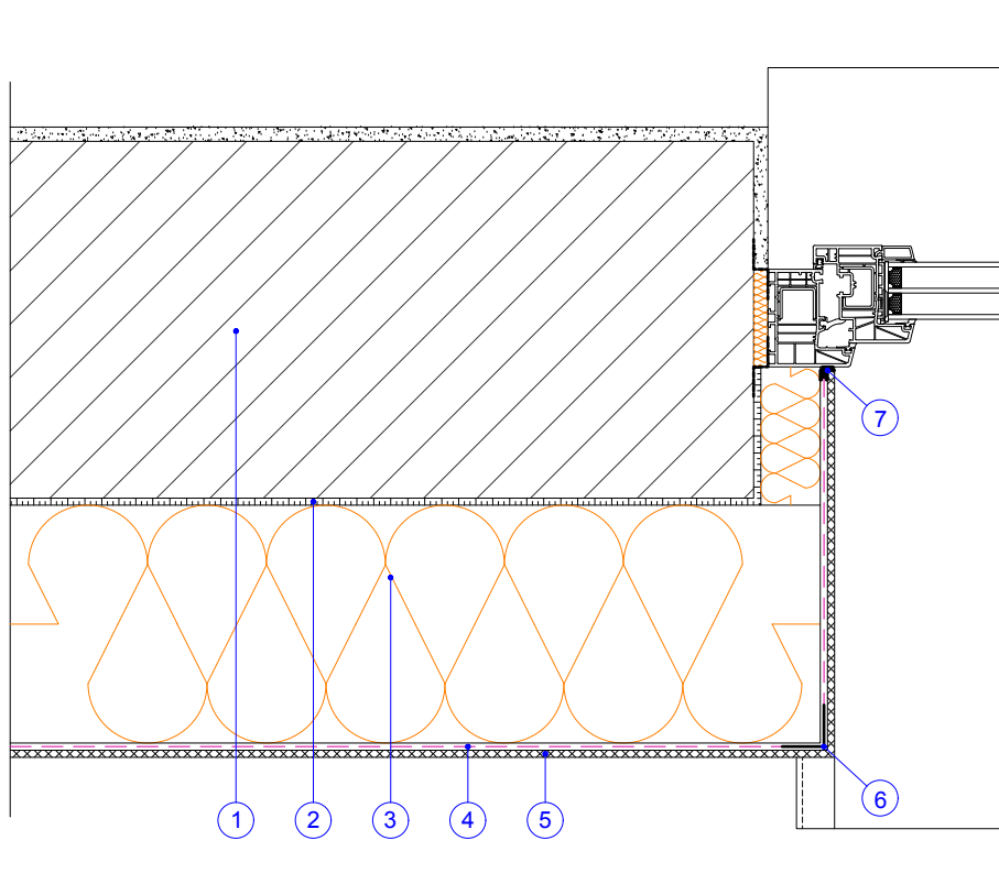
ALTERNATÍVA 1 okenná začistovacia lišta
