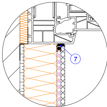
ALTERNATÍVA 1 okenná začistovacia lišta
