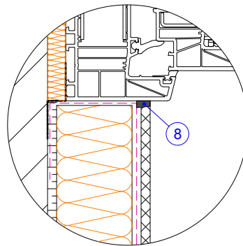
ALTERNATÍVA 2 zámok + pretierateľný pružný tmel
