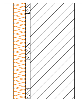
REZ B-B'
