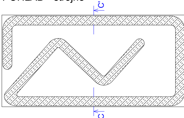
POHĽAD - strojne
